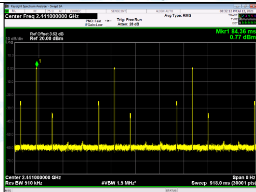
2441MHz DH5
