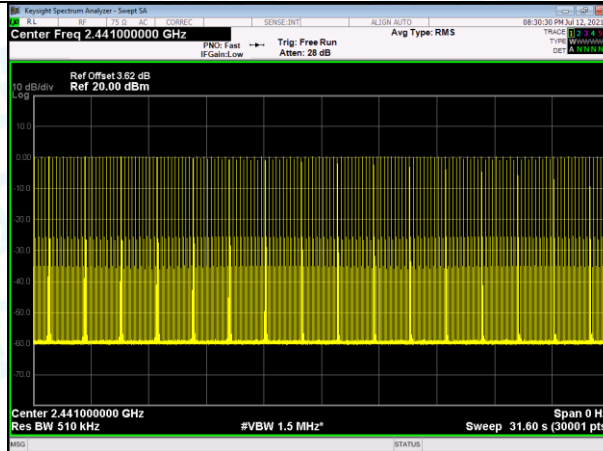
2441MHz DH5
