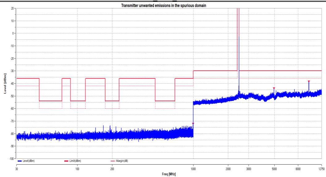
2DH5 Ant1 2480
