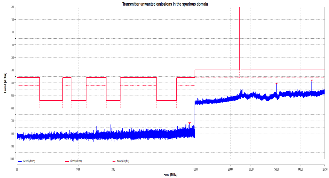
2DH5 Ant1 2402
